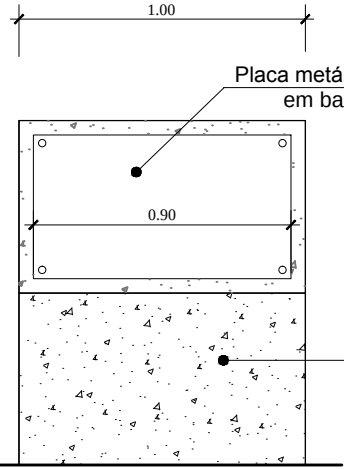
VISTA FRONTAL TOTEM ESC.1/25
