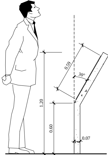
VISTA LATERAL TOTEM ESC.1/25
